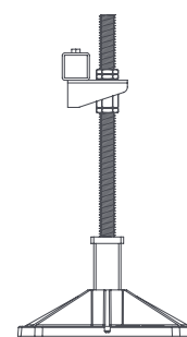
Komplettes Bein mit verlängerter Gewindestange Höhenverstellung: 335 - 660 mm
